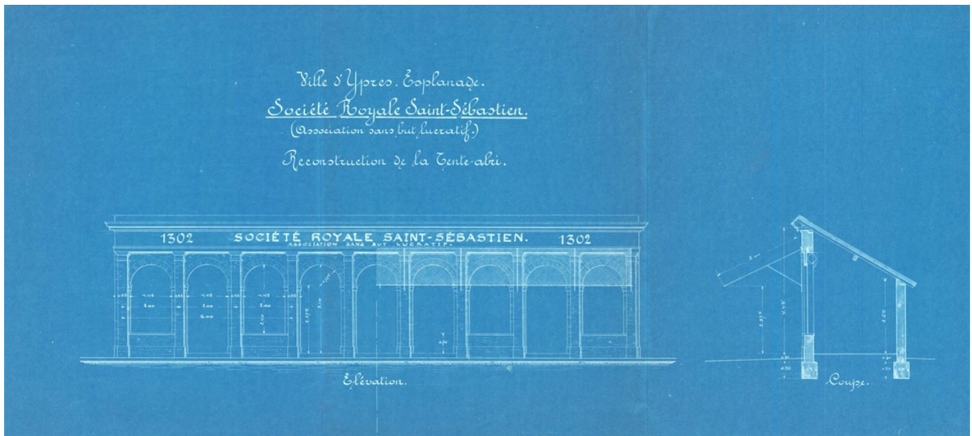
Heropbouwplan van het schutterslokaal van de Ieperse Sint-Sebastiaansgilde op de Esplanade na de Eerste Wereldoorlog. SAI, Sint-Sebastiaansgilde, 216.
